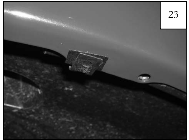
Install clip (SW1-0022) over 1"x1.5" Black Tab.
